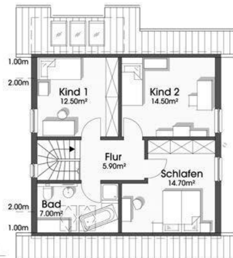
Dachgeschoss 1:175 54.40 m 2
