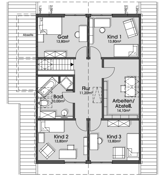
Dachgeschoss 1:150 90,50 m 2
