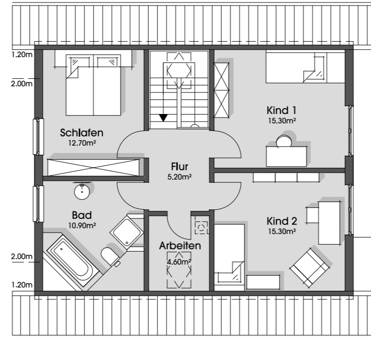
Dachgeschoss 1:125 64.00 m 2
