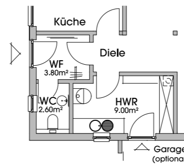
Erdgeschossvariante 1:150 Eingang im Giebel + Seiteneingang
